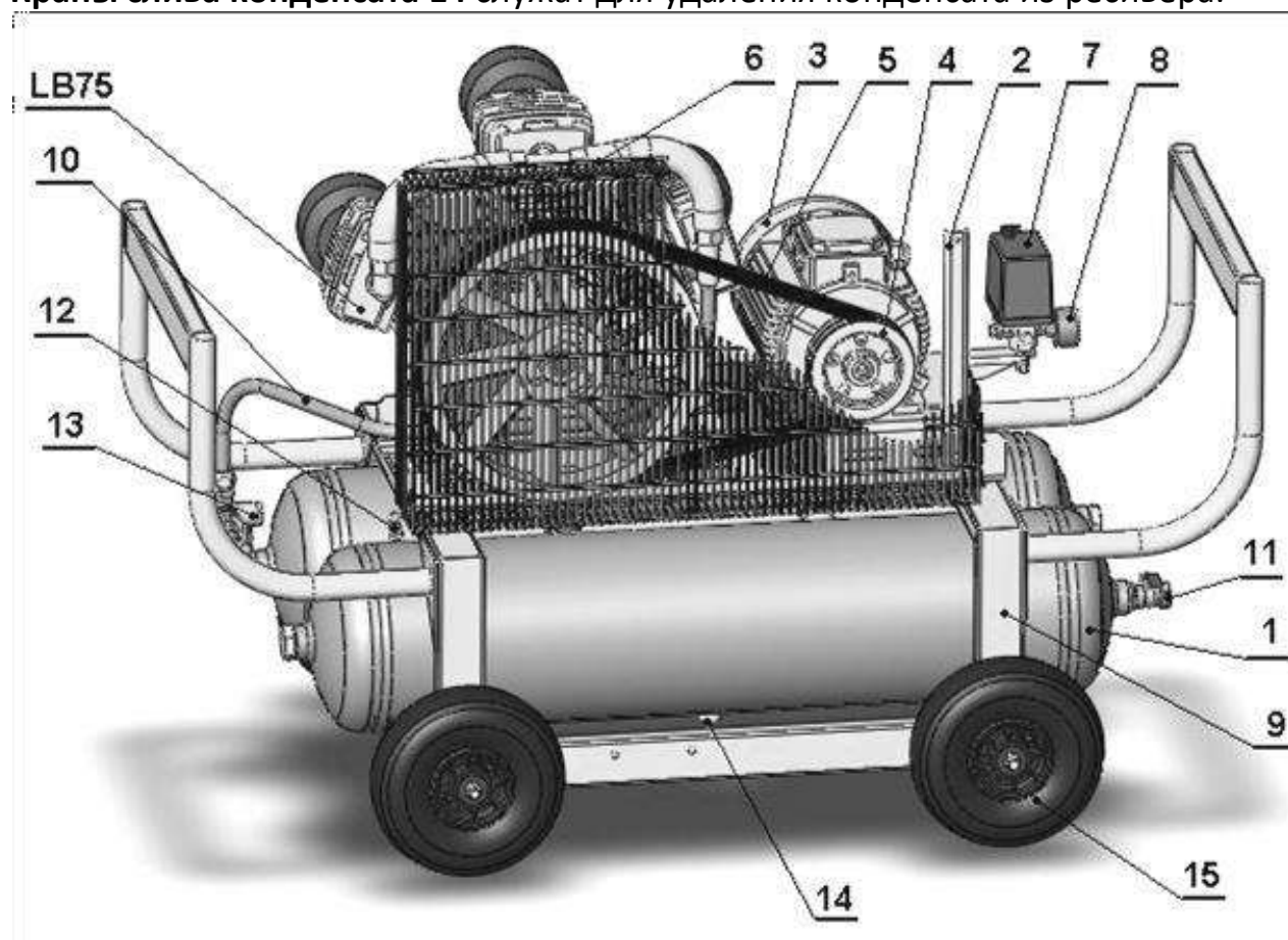
Рисунок 1 – Общий вид компрессора СБ4/С-90.ЛВ75
