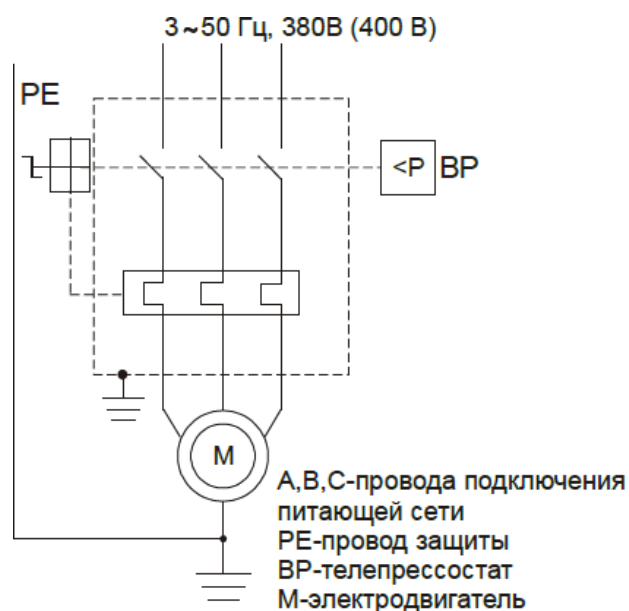
Рисунок 2 – Схема электрическая принципиальная
